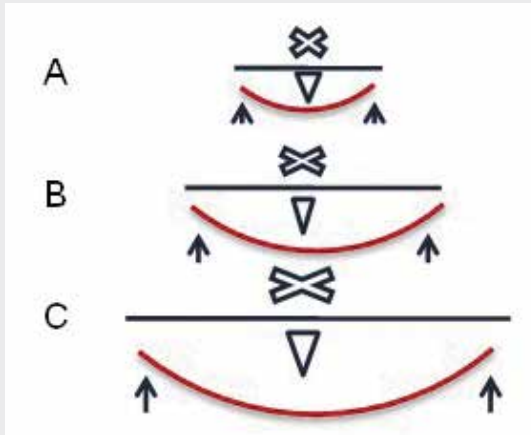
FIGURA N.º 8 LA FLEXIÓN DEL METAL ESTÁ RELACIONADA CON EL CUBO DE LA DISTANCIA DE A. CUANDO HAY UN PÓNICO EL METAL SE FLEXIONA X . B, CUANDO TIENE DOS PÓNICOS ( 2X ) EL METAL SE FLEXIONA 2 \times 2 \times 2 = 8 VECES MÁS. C, CUANDO EXISTEN TRES PÓNICOS ( 3X ) EL METAL SE FLEXIONA 3 \times 3 \times 3 = 27 VECES MÁS QUE UNA RESATURACIÓN DE UN PÓNICO.
